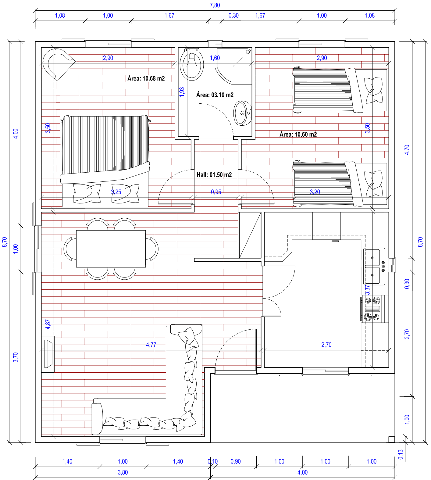
Planta do Piso Área: 61,86 m 2 (sem a entrada coberta)
