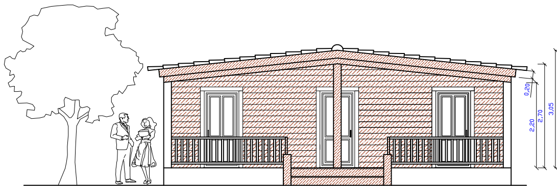
Alçado Principal
